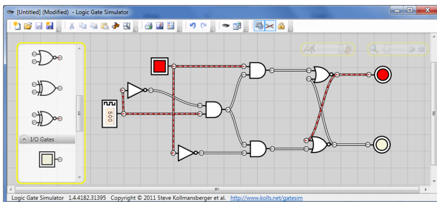
2-nji surat. D-triggeriň programmada wizuallaşdyrylyşy
