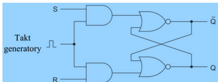
2-nji çyzygy. Sinhron SR -berkidiji
