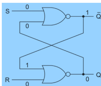
1-nji çyzgy. SR -berkidiji
