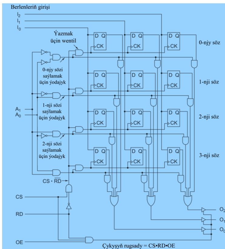
6-njy çyzgy. Uly göwrümlü ýat gurluşy
