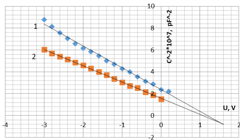
1-nji çyzygy. Au-n-Ga 1-x Al x As-n-GaAs 1-x P x Şottki diodynyň sygymynyň (C)naprýażeniýe (U) baglylygynyň C -2 -U koordinatada gurlan grafigi (1- S=3,5·10 -2 sm 2 ; 2- S=7,5·10 -2 sm 2 )
