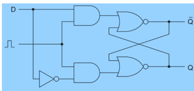
3-nji çyzygy. Sinhron D -berkidiji
