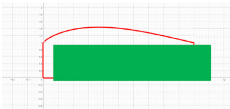
1-nji surat. Berlen kesgitli integralyň (gyzyl reňkli figura) we onuň n = 1 bolandaky takmyny bahasy (ýaşyl reňkli gönüburçluk)
