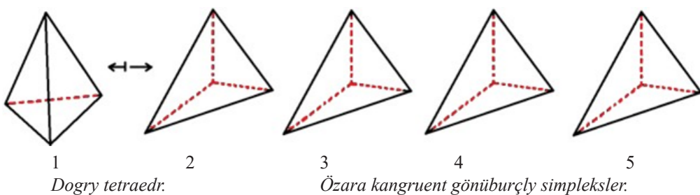
6-njy surat. Geksaedrden kesip alnan simpleksler
