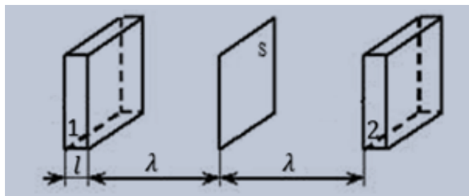
1-nji surat. S üstden geçýän molekulalaryň hereketiniň ugurlary
