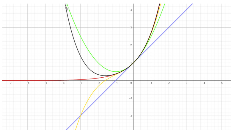
1-nji surat. Eksponensial funksiýanyň we oňa ýakynlaşan funksiýalaryň grafikeleri
