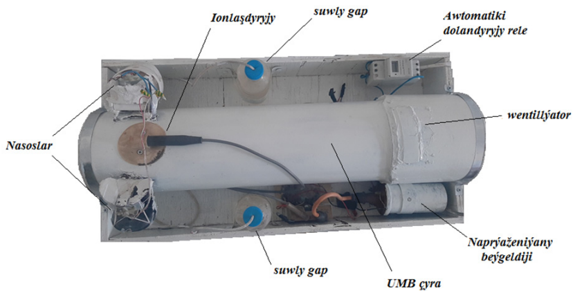
2-nji surat. Kondensirlenen zyýansyzlandyryjy-ionizator
