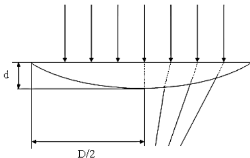
1-nji surat. Tekiz-güberçek linzadan şöhläniň geçişi. Bu ýerde D – linzanyň diametri, d – linzanyň galyňlygy
