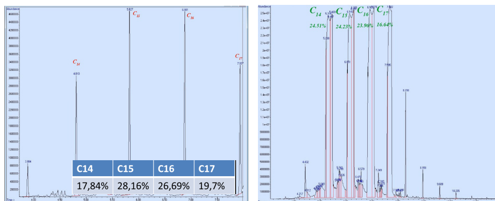
3-nji surat. Göni kowgy edilen agyr benziniň düzüminden bölünip alnan n-parafinler hromatografiki analiz netijesi
