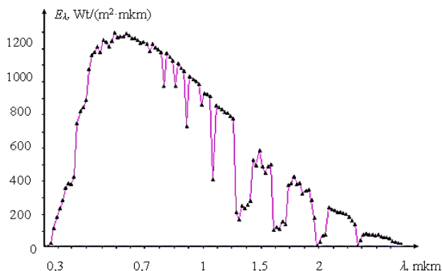
2-nji surat. Gün radiasiýasynyň akymynyň spektral dykzlygynyň onuň tolkun uzynlygyna baglylygynyň grafigi
