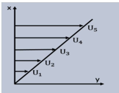
2-nji surat. Gatlar boýunça gaz molekulalarynyň tizliginiň üýtgeşi
