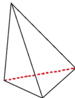
3-nji surat: (üç ölçegli simpleks)
