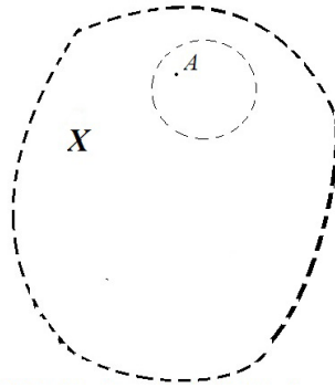
2-nji surat. ( X köplügiň açyk köplük bolmagynyň şertiniň geometrik mazmuny)
