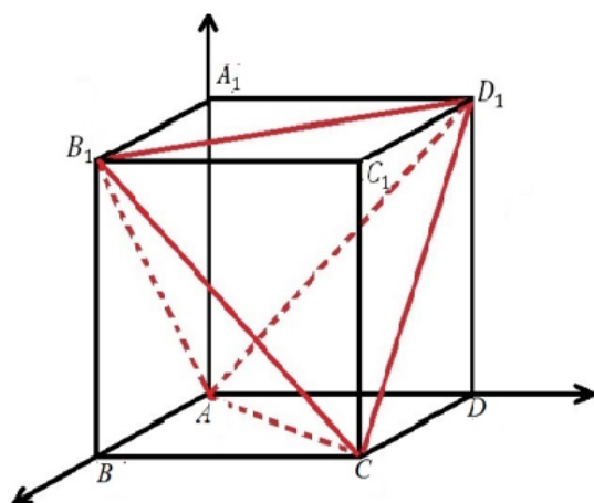
4-nji surat. Dogry geksaedr
