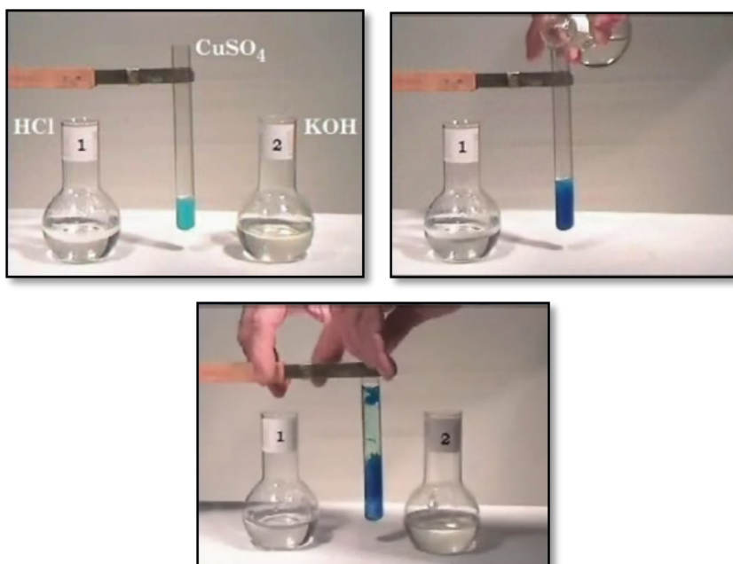
1-nji surat. Mis (II) gidroksidiniň alnyşy we häsiýetleri
