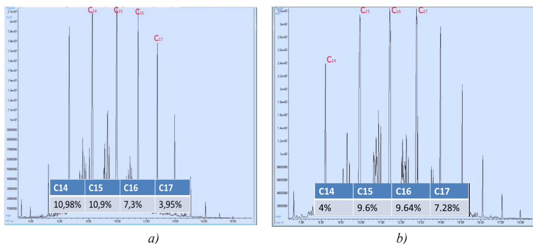
2-nji surat. Tagtabazar (a) we Sarahs (b) gaz kâniniň gazkondensatларыnyň karbamid bilen işlenenden soň alnan hromatografiki analiz netijeleri
