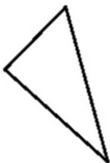
2-nji surat: (iki ölçegli simpleks)
