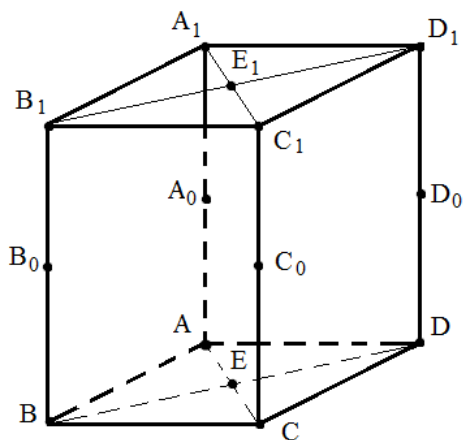
7-nji surat. F kompleksiň simplekslere bölünişi
